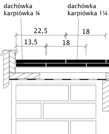
Rysunek techniczny produktu AMBIENTE KRÓJ SEGMENTOWY - przekrój poprzeczny połaci dachu
