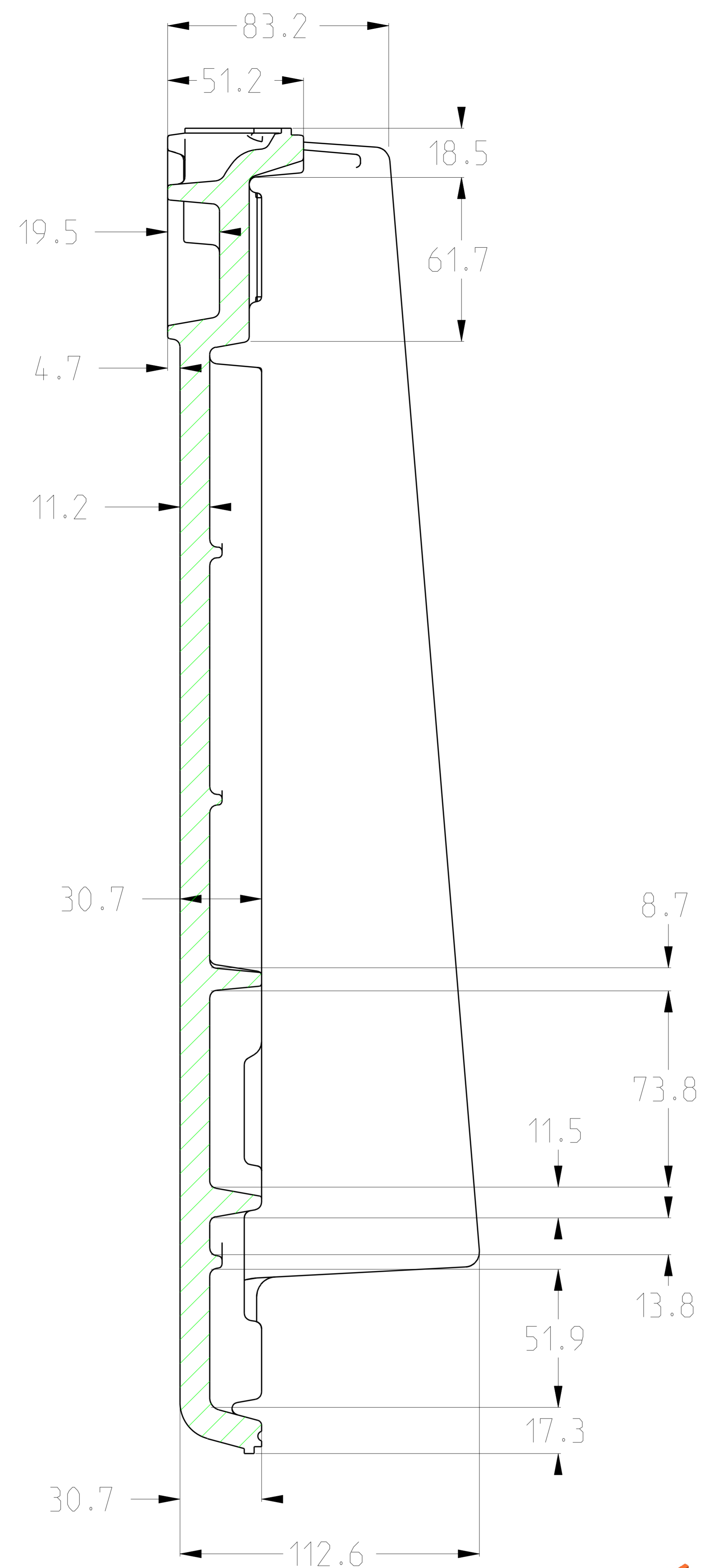
SECTION A-A
