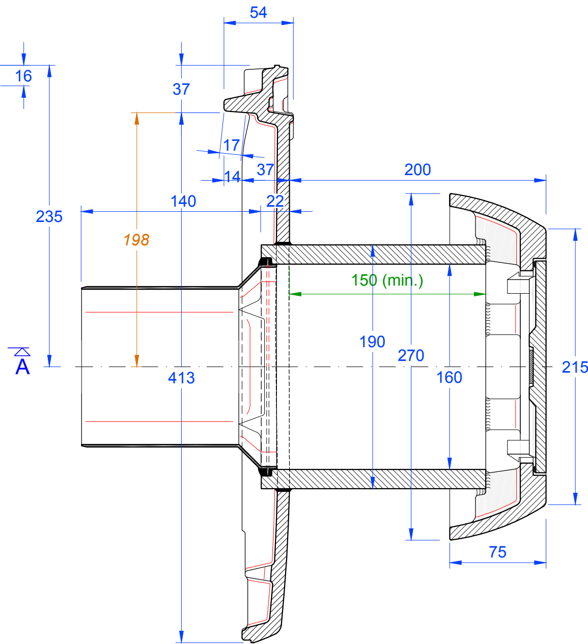
Schnitt B-B
