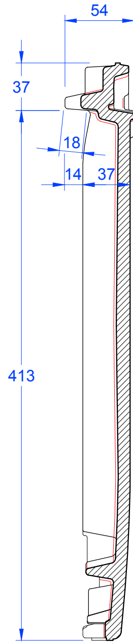
Schnitt B-B
