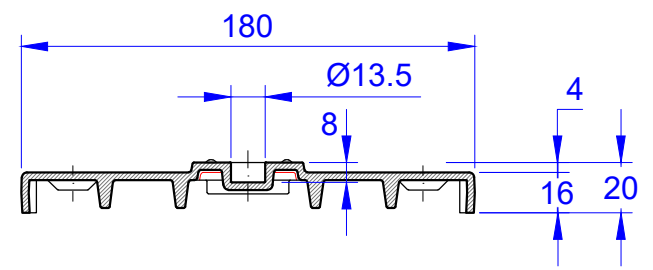
Schnitt A-A
