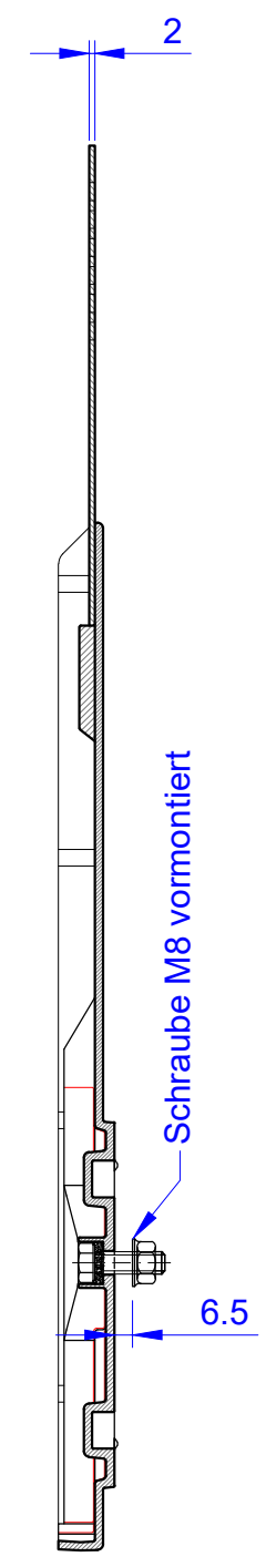
Schnitt B-B
