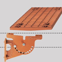
Ława kominarska aluminiowa długa 80/25 Ława kominarska aluminiowa krótka 46/25
