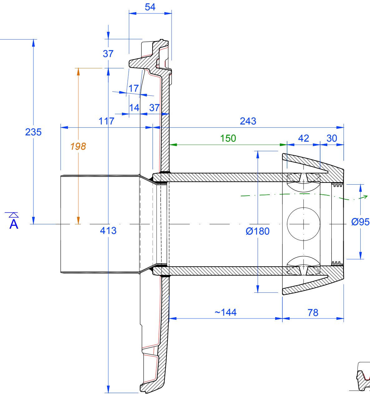
Schnitt B-B (ohne Deckel)
