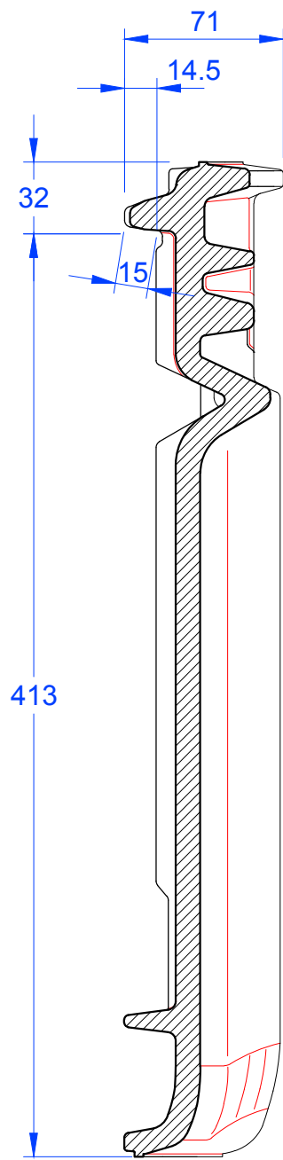
Schnitt B-B
