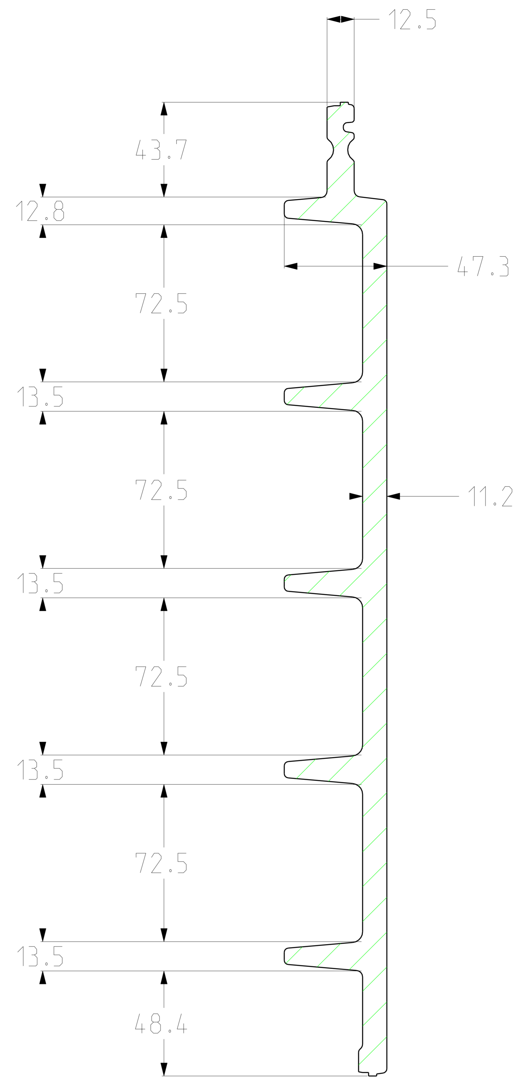
SECTION A-A
